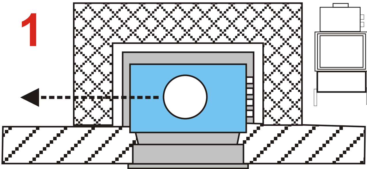
Glastüre 55 b x 44 h Wohnzimmerseite
