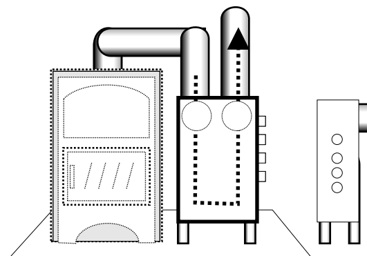
Seitlich angebautes Standregister Rauch Ein/Ausgang Rückseite (oben) Wasser rechte Seite
