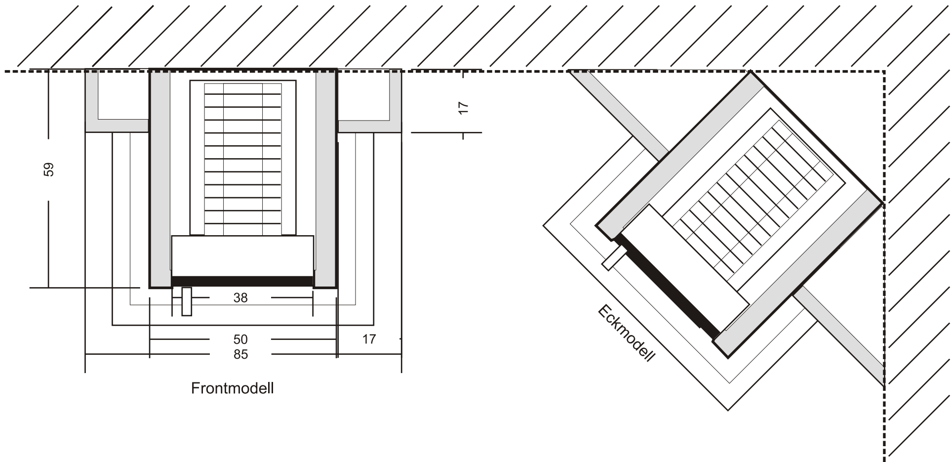
Grundriss-Plan M= 1:10 Modell Landshut Mini 1 für ein oder zwei Wasserregister Nennwärmeleistung 15 oder 21 kW
