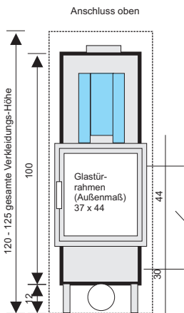
Einsatz: 37x44, +8 Verkleidung 125
