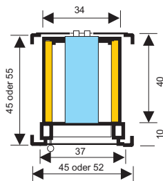
Einsatz: 37x44, +8 Verkleidung 125
