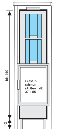
Einsatz: 37x55, +8+8 Verkleidung 160
